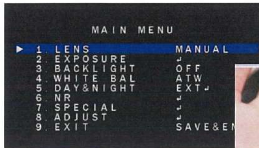
◆ケーブル一体型リモコンでOSD操作
